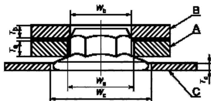
A — калибр A ; B — калибр B ; C — калибр C
