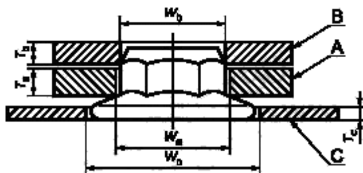
Рисунок А.1 — Схема контроля шестигранника и фланца
