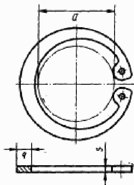
Кольцо, скатанное для установки
