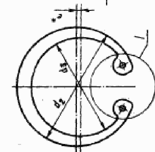
Кольцо в свободном состоянии
