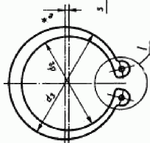
Кольцо в свободном состоянии
