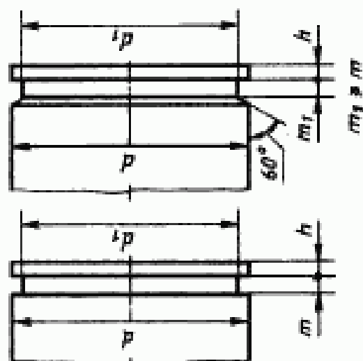
Вариант исполнения канавки при односторонней осевой нагрузке
