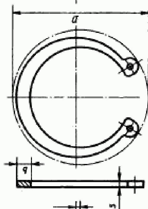
Кольцо, разведенное для установки
